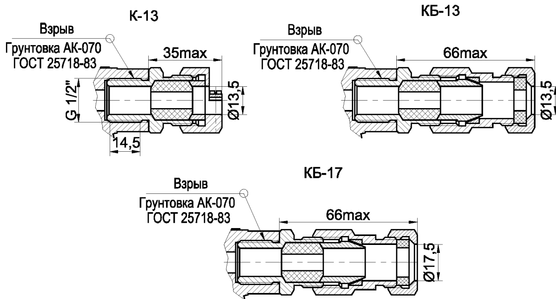
Рисунок А.7 – Перечень рекомендуемых кабельных вводов
