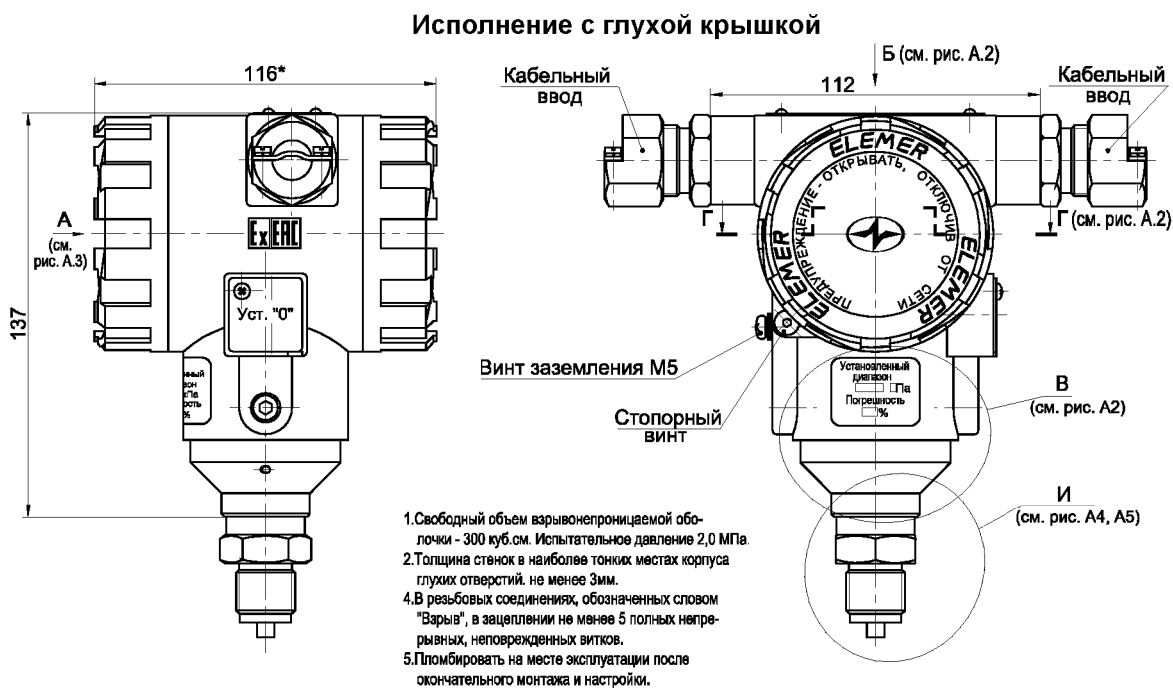
Рисунок А.2 – Чертеж средств взрывозащиты
