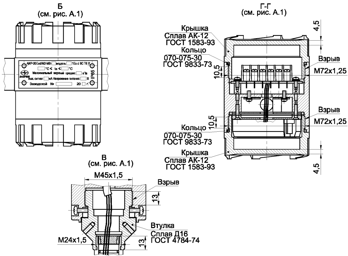
Рисунок А.3 – Чертеж средств взрывозащиты
