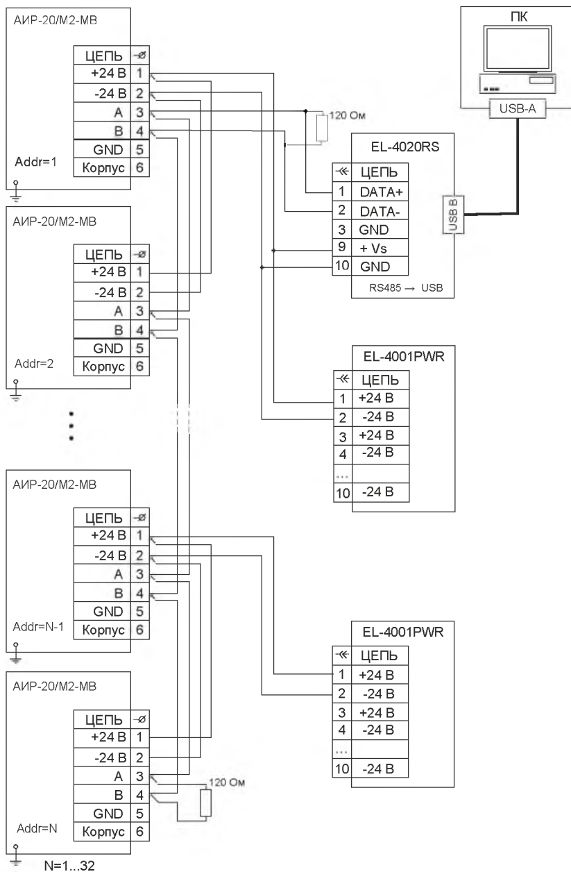
Рисунок 3.2 – Схема электрическая сетевого подключения АИР-20/М2-МВ (исполнение с кабельными вводами)
