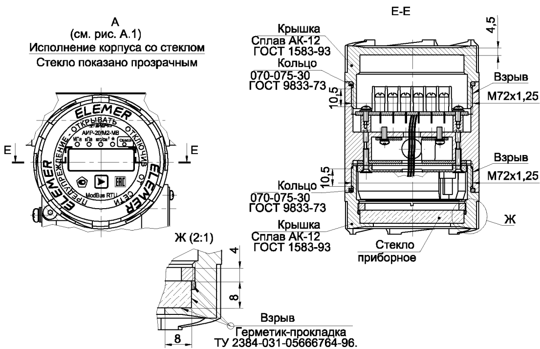
Рисунок А.4 – Чертеж средств взрывозащиты
