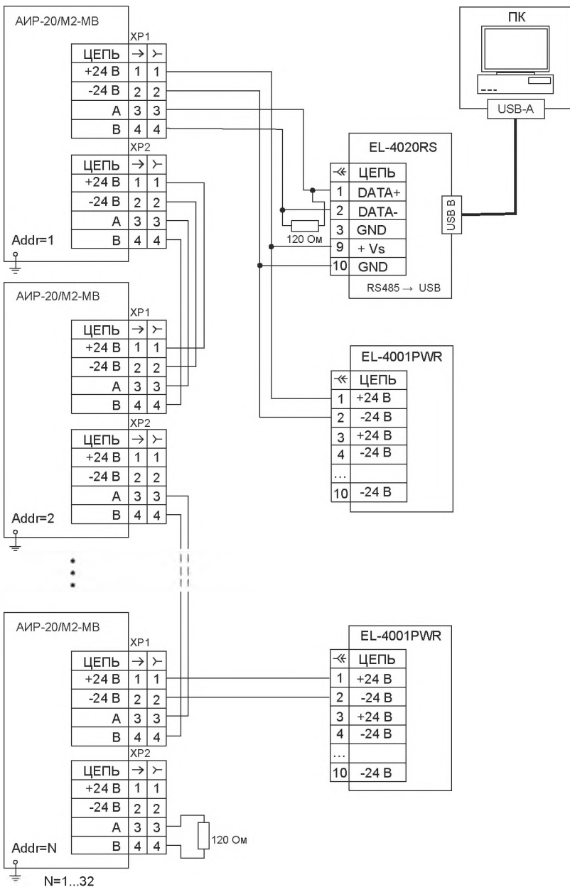
Рисунок 3.1 – Схема электрическая сетевого подключения AIР-20/M2-MВ (исполнение с разъемами)
