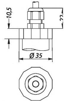
Кабельный ввод (IP 67) 1,2
