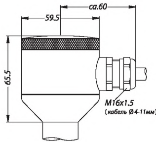
Binder 723 (IP 67)
