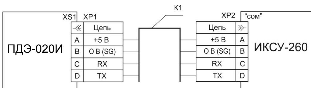
Рисунок 3 - Схема внешних электрических подключений преобразователя к ИКСУ-260, ИКСУ-260L или «ИКСУ-2012»
