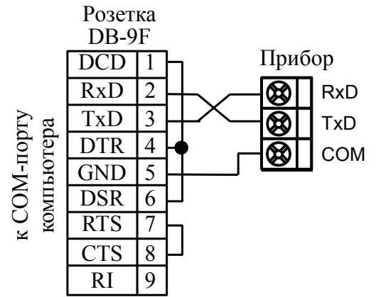
Рисунок Г.6 - Подключение прибора настенного исполнения с интерфейсом RS-232 к COM-порту компьютера
