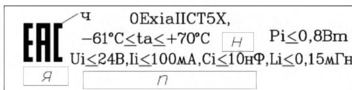
Вид Ф
