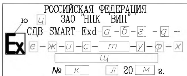
Вид Г
