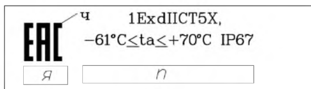
Вид И
